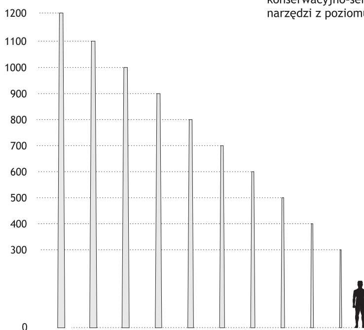
Dostępne wysokości słupów kompozytowych na fundamencie
